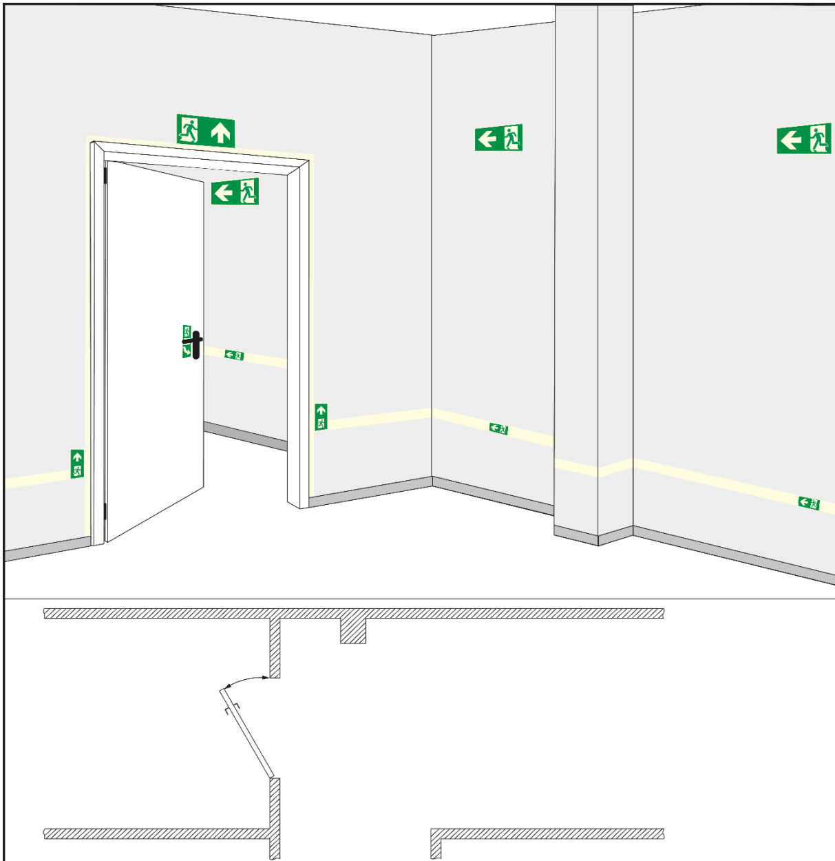
Abb. 1: Beispiel für die Anordnung von Komponenten eines langnacheuchtenden optischen Sicherheitsleitsystems und hochmontierter langnacheuchtender Sicherheitszeichen (räumliche Darstellung und Grundriss)
